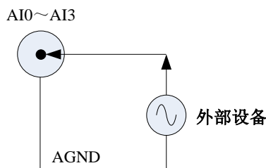
图 4-4-1 AD 信号连接
