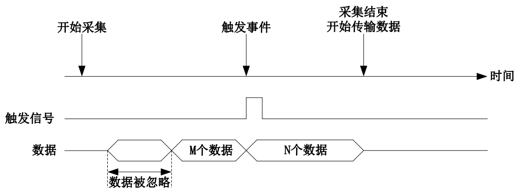
图 4-10-2 中间触发
