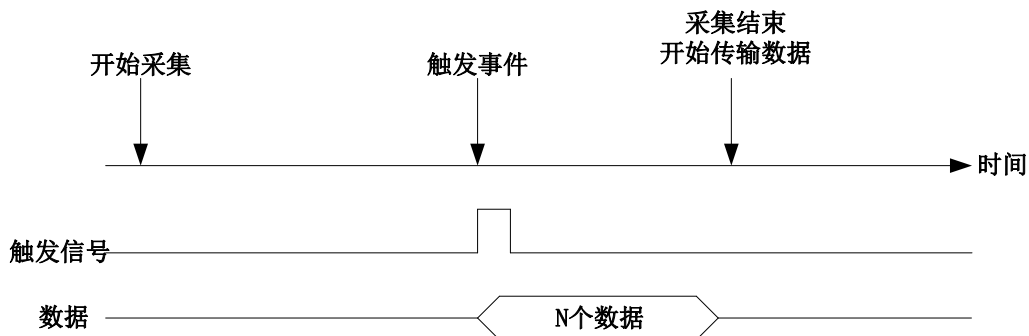
图 4-10-3 后触发
