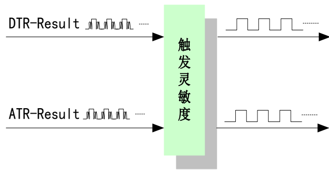
图 4-9-2 触发灵敏度
