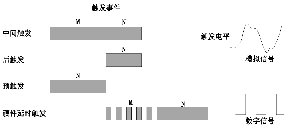
图 4-10-1 AD 触发模式
