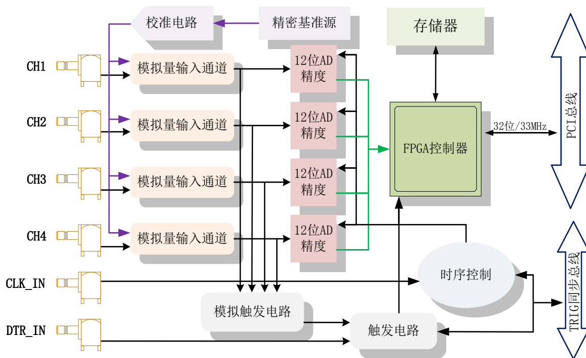
图 3-1-1 PCI8502B/8512B 系统框图
