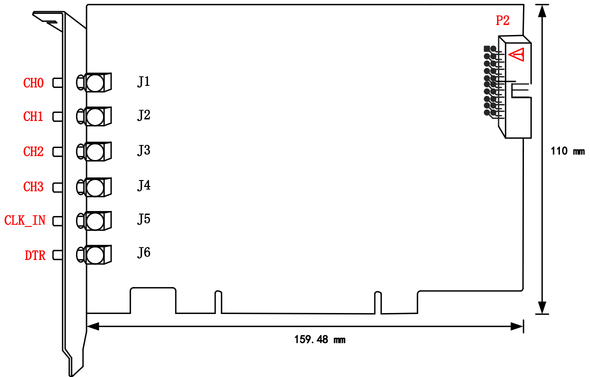
图 3-2-1 PCI8502B/8512B 板卡尺寸图
