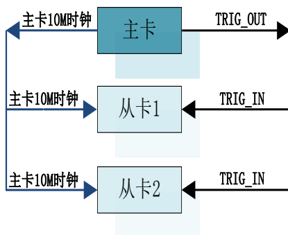
图 4-11-1 主从卡级联
