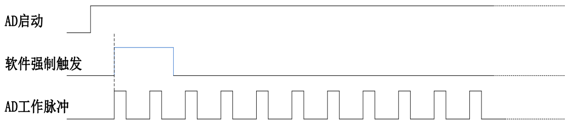
图 4-9-3 AD 软件触发
