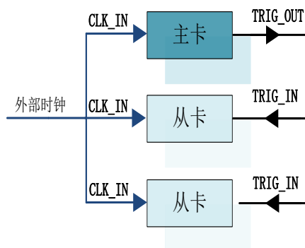
图 4-11-2 采用共同外时钟
