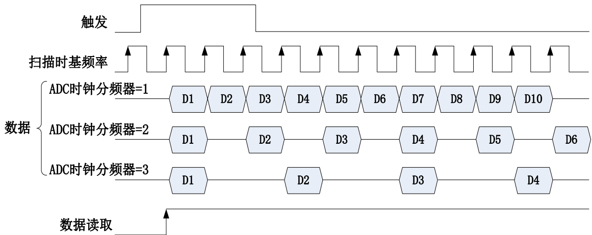
图 4-7-2 AD 抽样速率示意图
