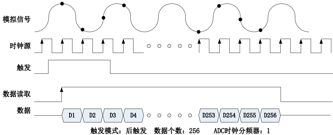
图4-8-1 AD后触发采集示意图
