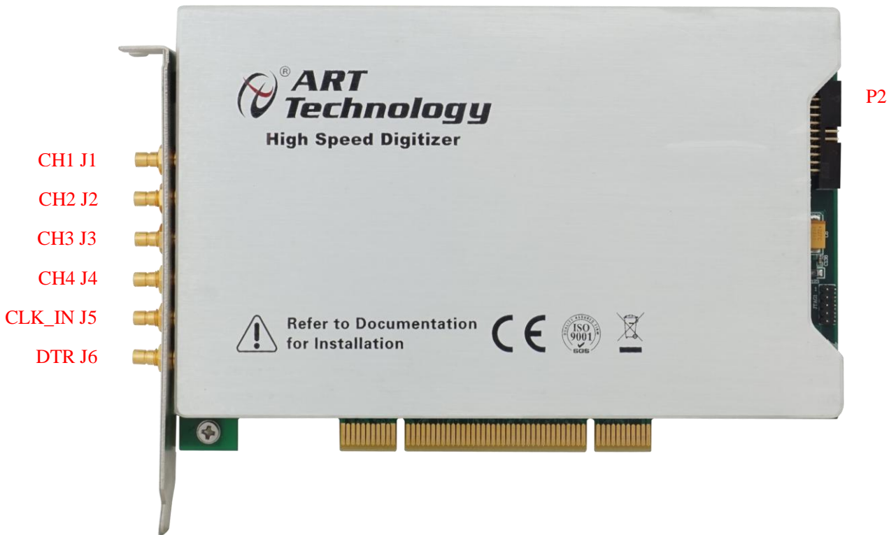
图 3-3-1 PCI8502B/8512B 元件布局图
