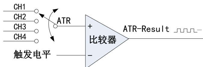
图 4-9-5 比较器
